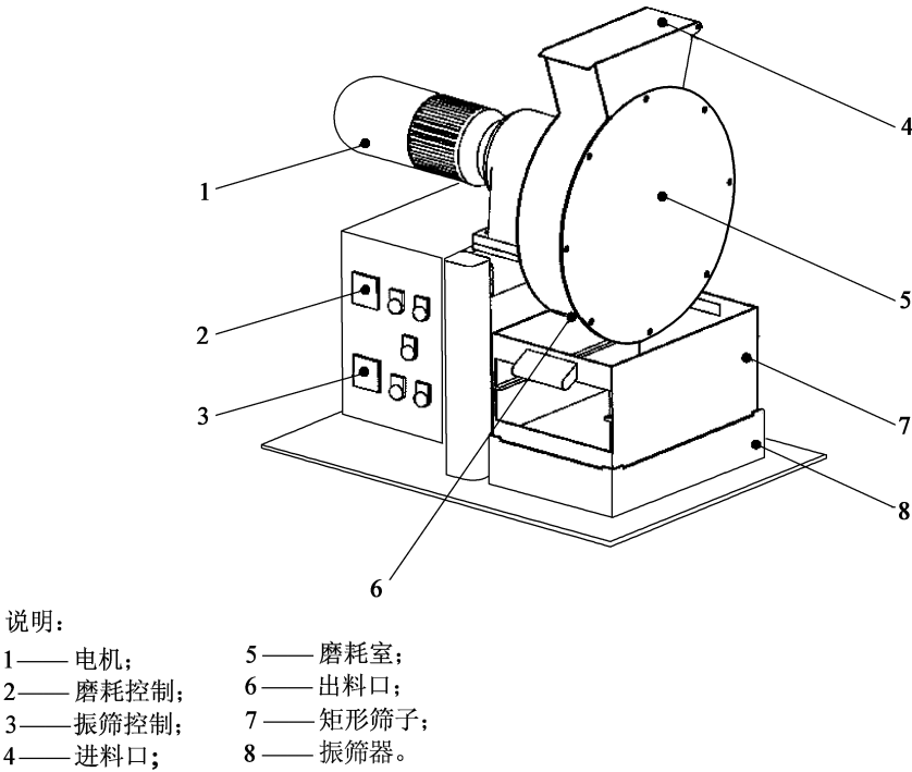
图 L.1 纤维磨耗机结构示意图
