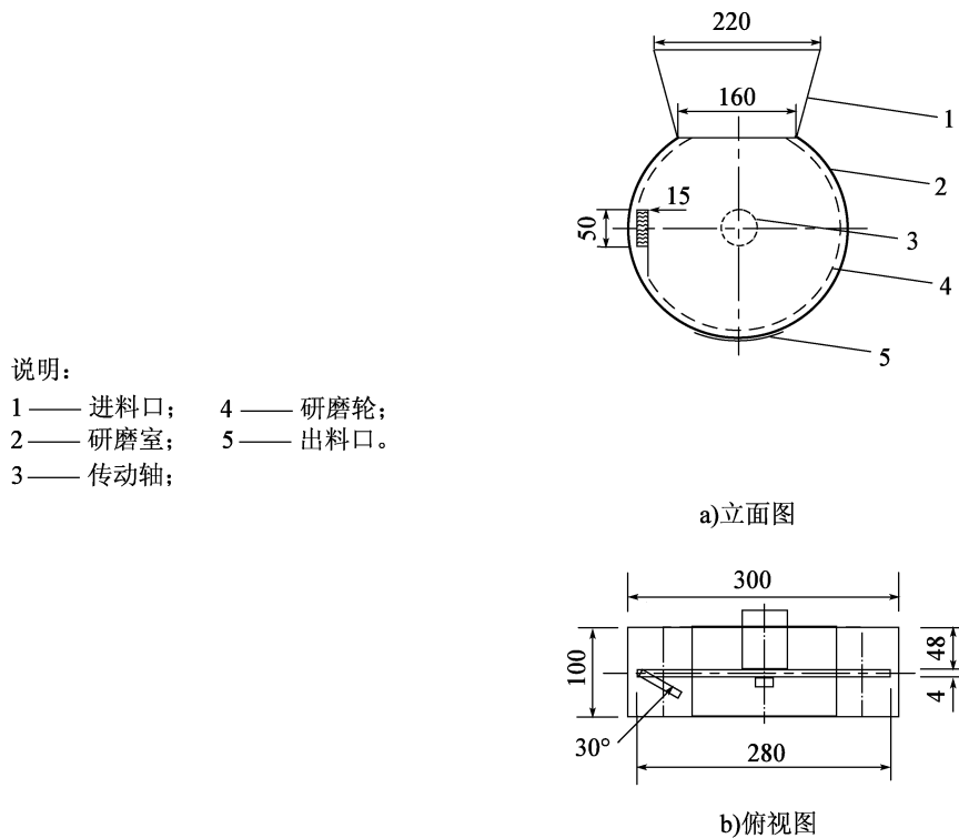
图 L.2 研磨系统结构示意图(尺寸单位:mm)
